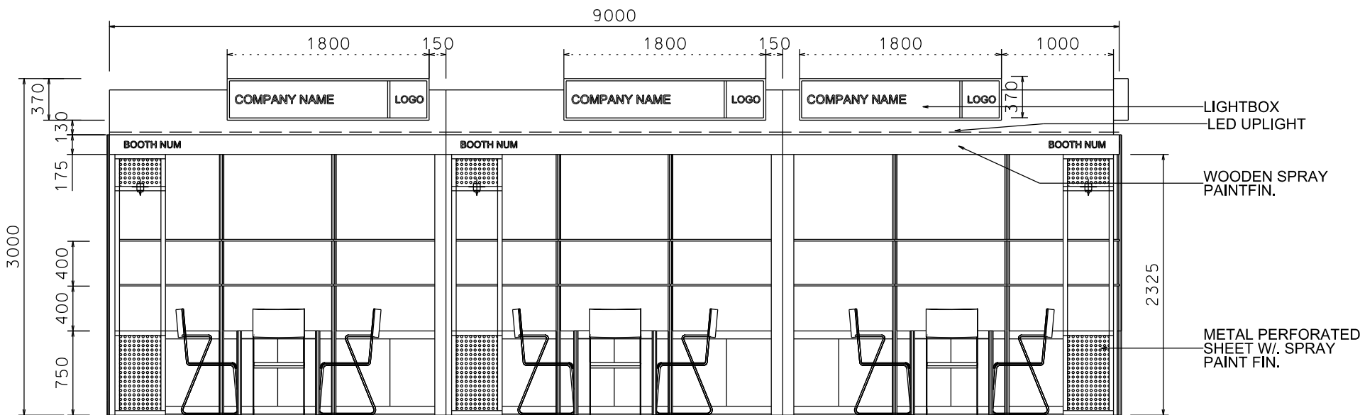
ELEVATION
