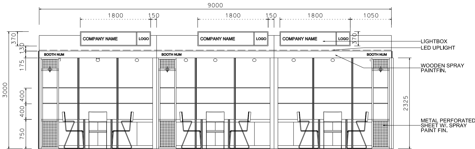
ELEVATION
