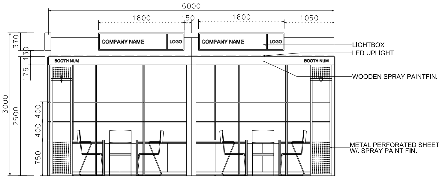
ELEVATION
