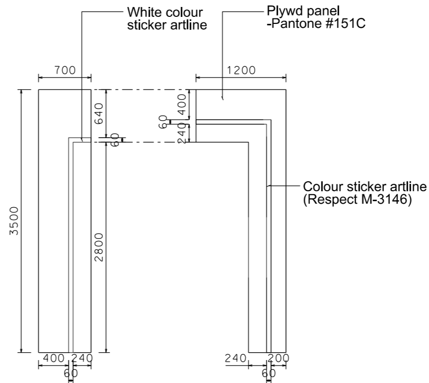
FASCIA ELEVATION
