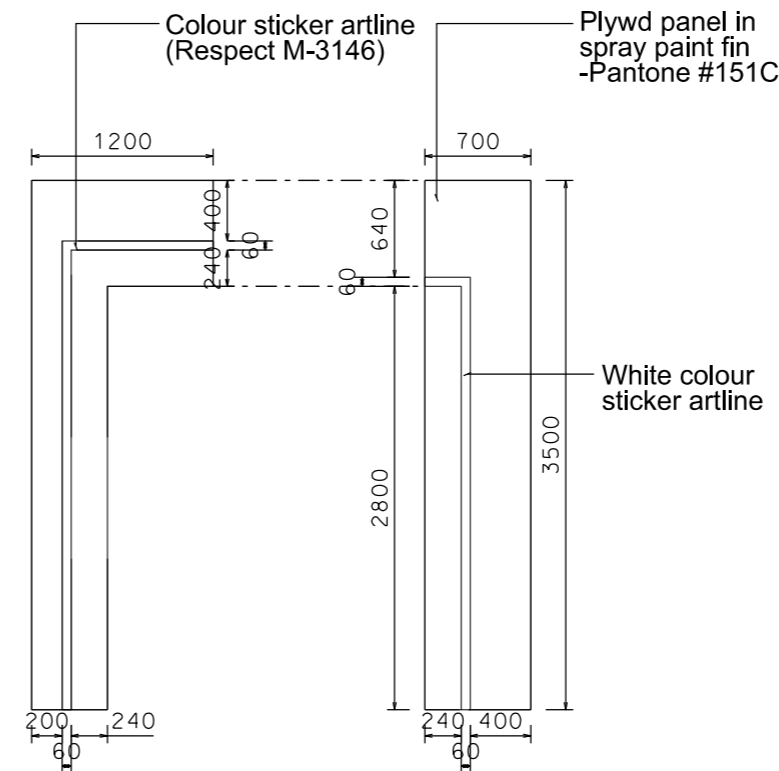
FASCIA ELEVATION
