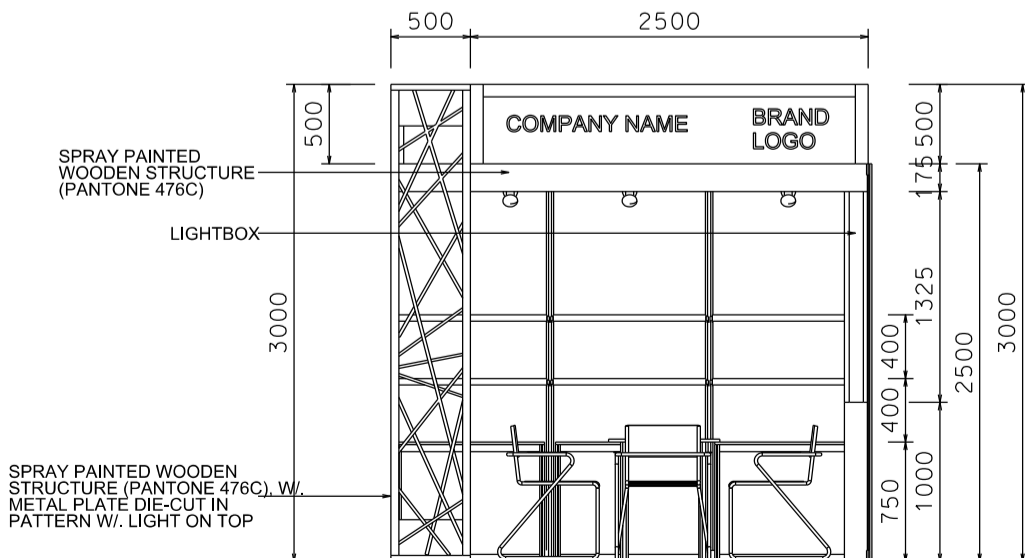
ELEVATION
