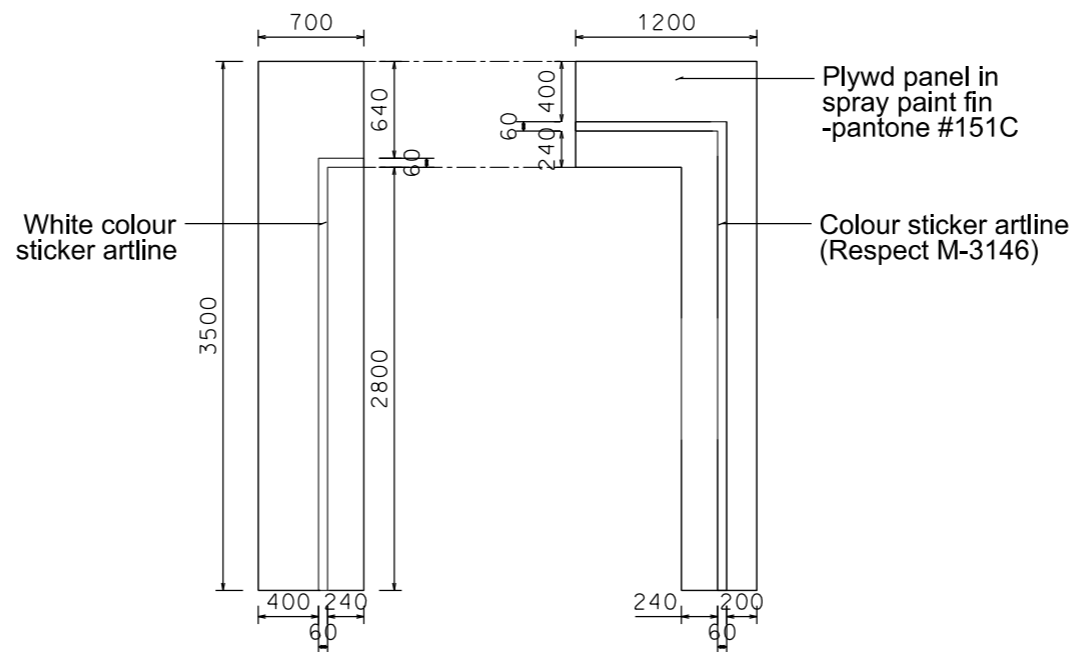
FACSLA ELEVATION
