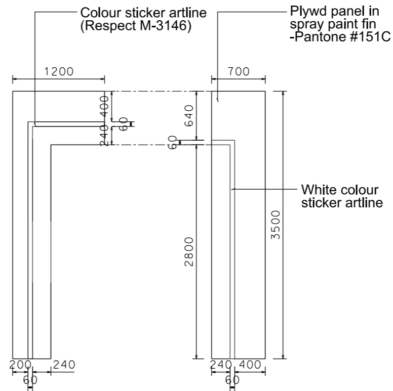
FACسيا ELEVATION
