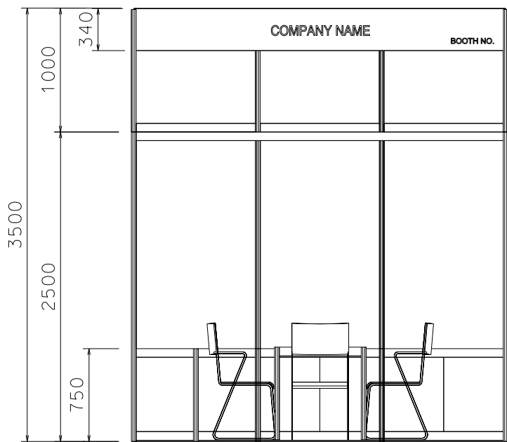
ELEVATION 3M(W) X 3M(D) X 3.5M(H)
