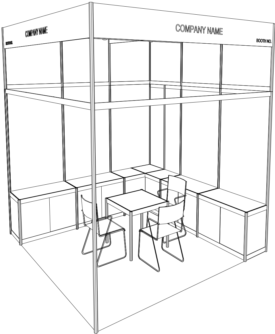
PERSPECTIVE 3M(W) X 3M(D) X 3.5M(H)
