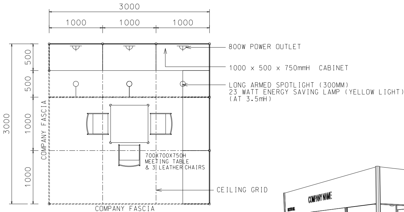
PLAN 3M(W) X 3M(D) X 3.5M(H)
